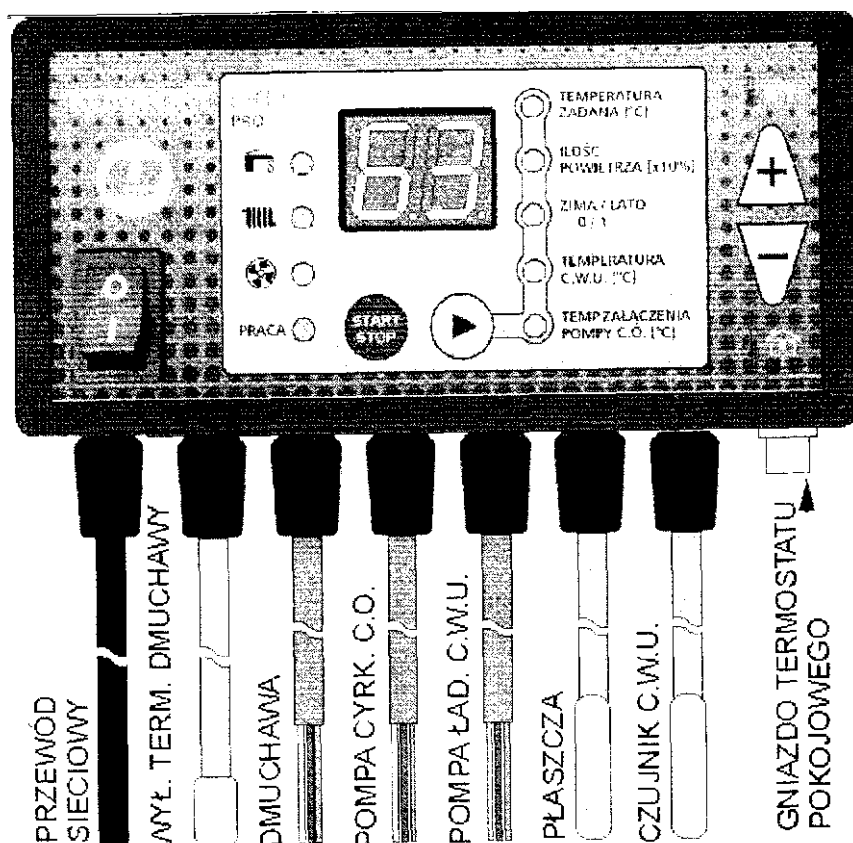
Рис.2. Выведения проводов и датчиков из корпуса регулятора
